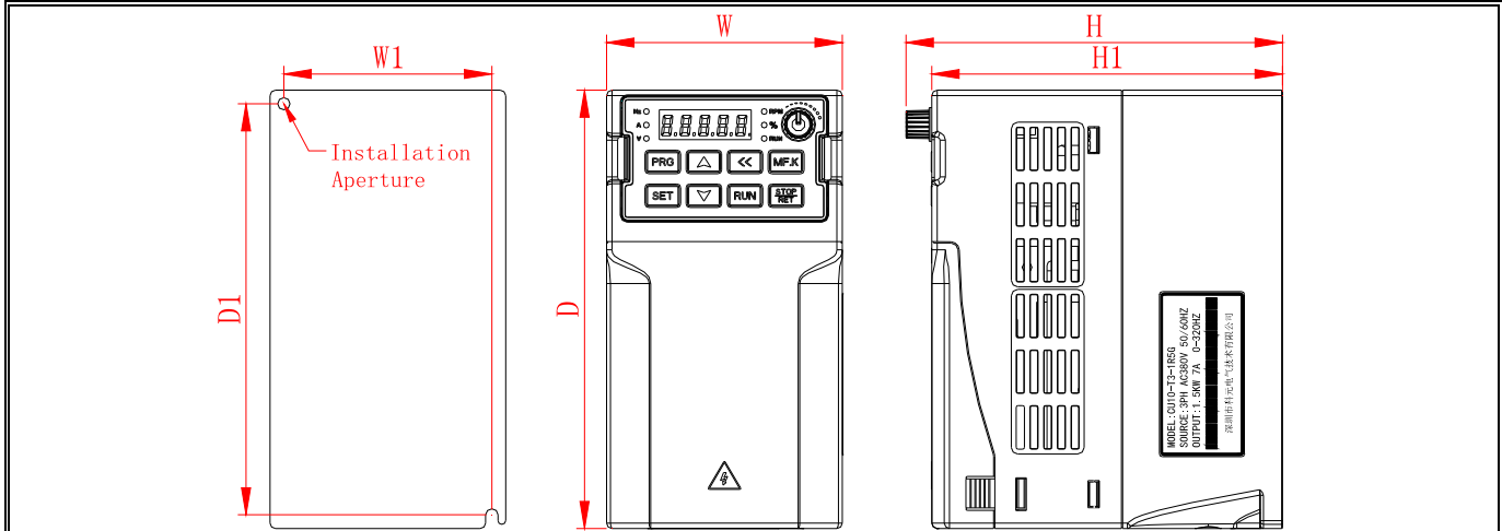
SV10 0.75G-4G 外型及安装孔位尺寸
