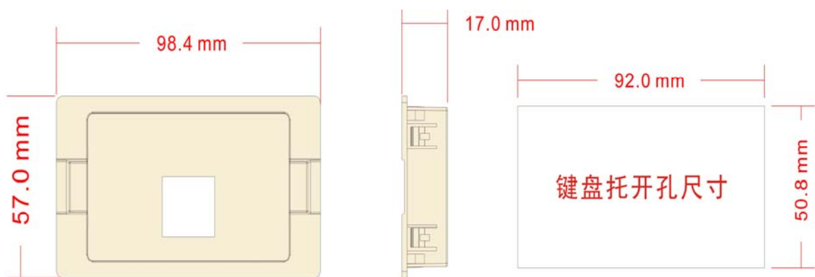
SV10 系列外引键盘外形尺寸
