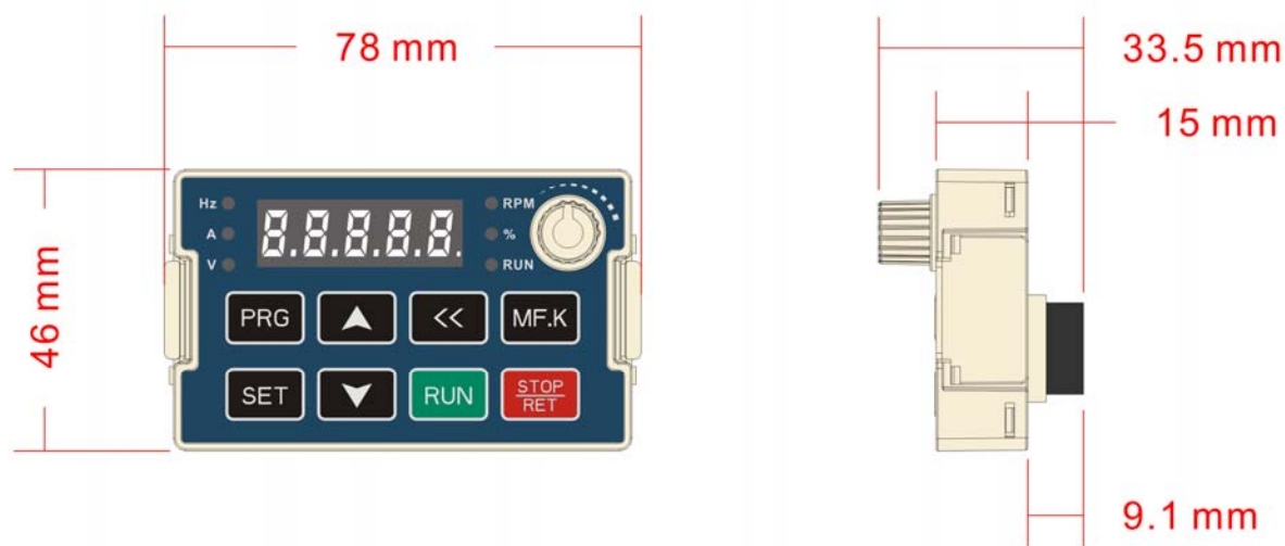
SV10 系列外引键盘外形尺寸
