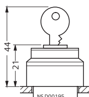
RONIS钥匙开关
