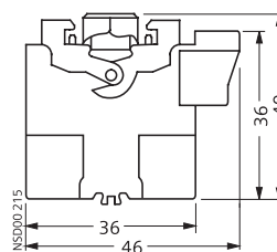
带灯按钮 带单触点块和灯座
