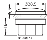
孔塞
