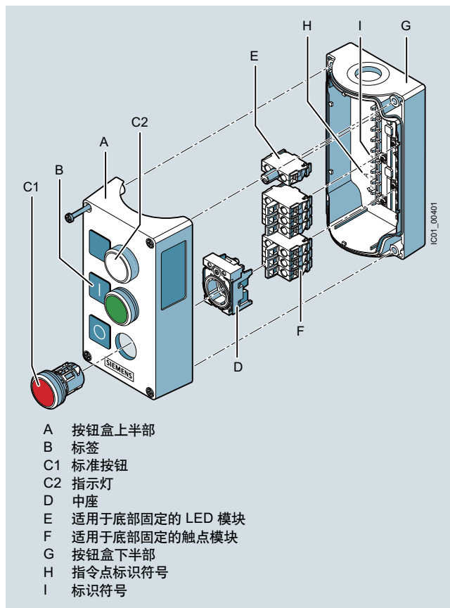
按钮盒内的按钮和指示灯
