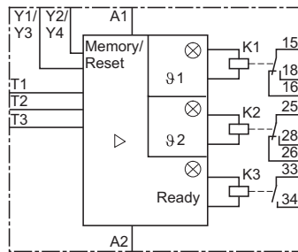
接线图
