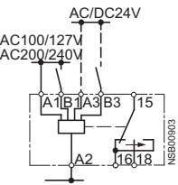
带辅助电压的脉冲成形
