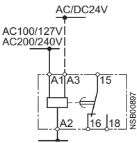
通电延时
