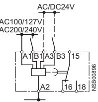
带辅助电压的断电延时
