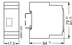
17.5 mm 结构
