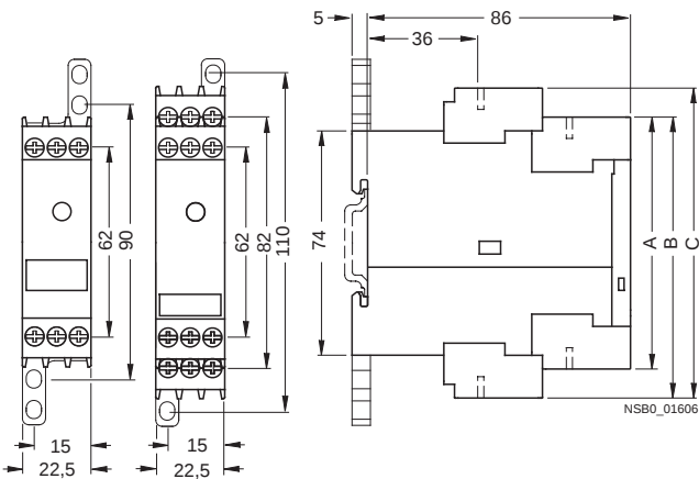
尺寸图 (单位: mm)
