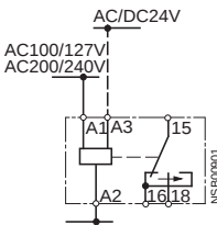
短时接通
