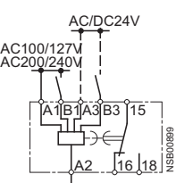
带辅助电压的通、断电延时
