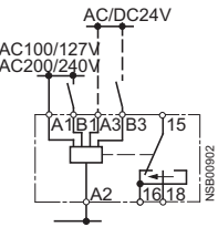
带辅助电压的短时接通
