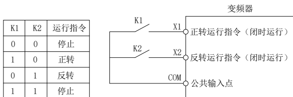
0:两线制控制1示意图
