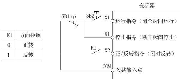
2:三线制控制1示意图
