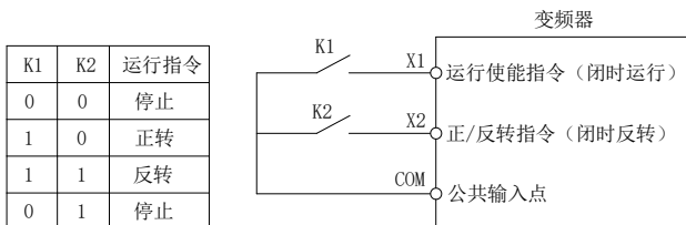
1:两线制控制2示意图
