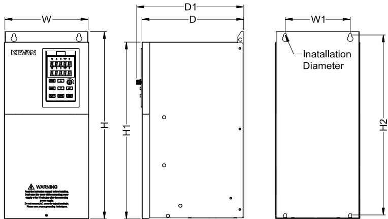
SV20 30G-400G 外型及安装孔位尺寸
