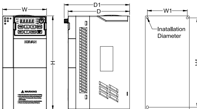
SV20 0.75G-22G 外型及安装孔位尺寸
