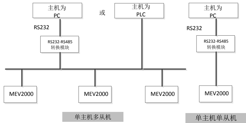
附图 4 变频器组网方式示意图
