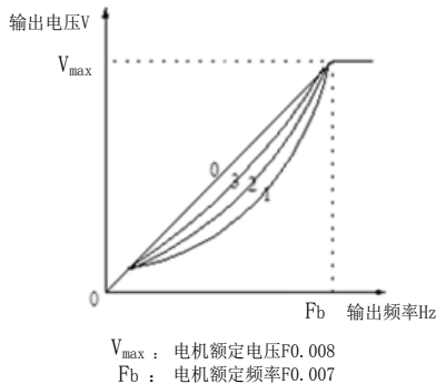
图 5-2 降转矩曲线
