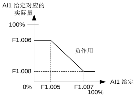
图5-7 模拟输入AI1给定反作用特性
