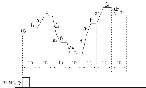
图 5-59 PLC 单循环后保持方式
