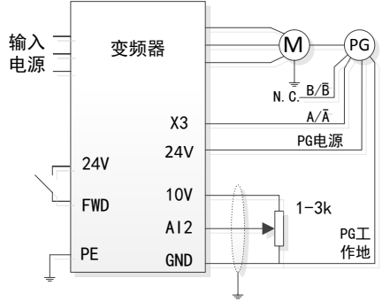
图 5-23 PG 速度闭环控制系统接线图
