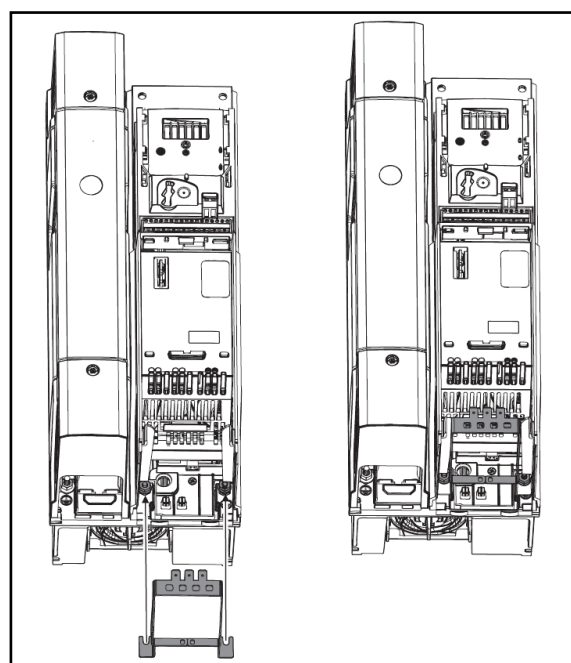
图 3-29 Size5-8 接地支架安装示意图（size5 为例）
