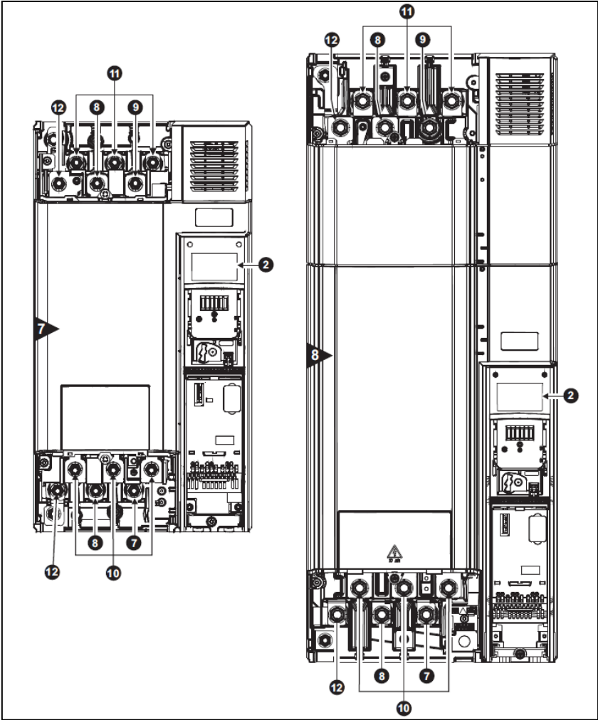
图 2-3 Size 7~8 变频器各部位名称示意图
