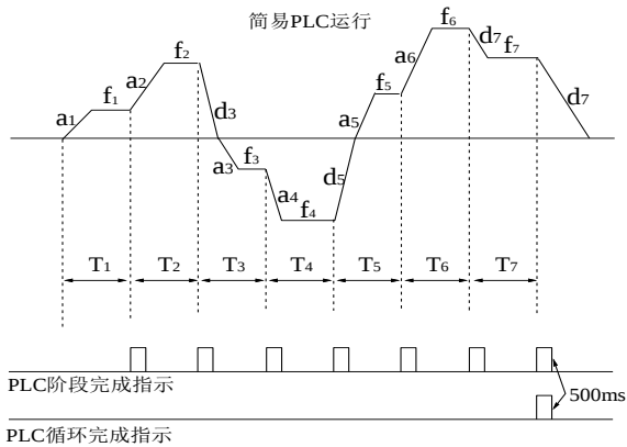
图 5-56 简易 PLC 运行图
