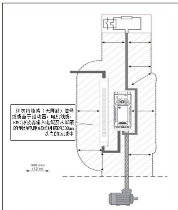
图 3-37 变频器线缆间隔
