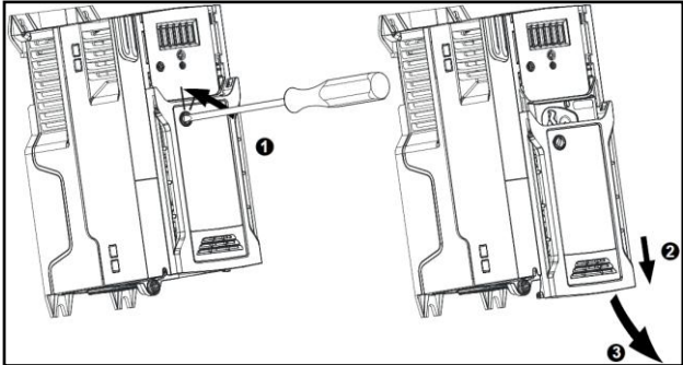
图 3-2 size2 ～ 4 盖板拆卸示意图
