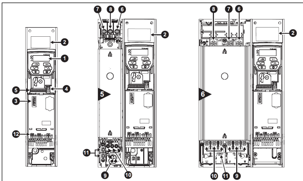
图 2-2 Size 5~6 变频器各部位名称示意图
