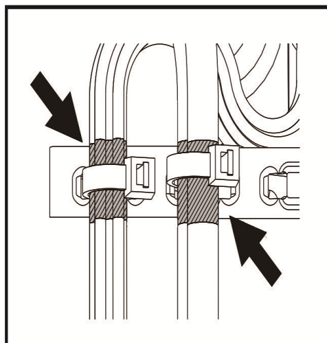
图 3-44 使用接地支架进行信号线缆屏蔽接地
