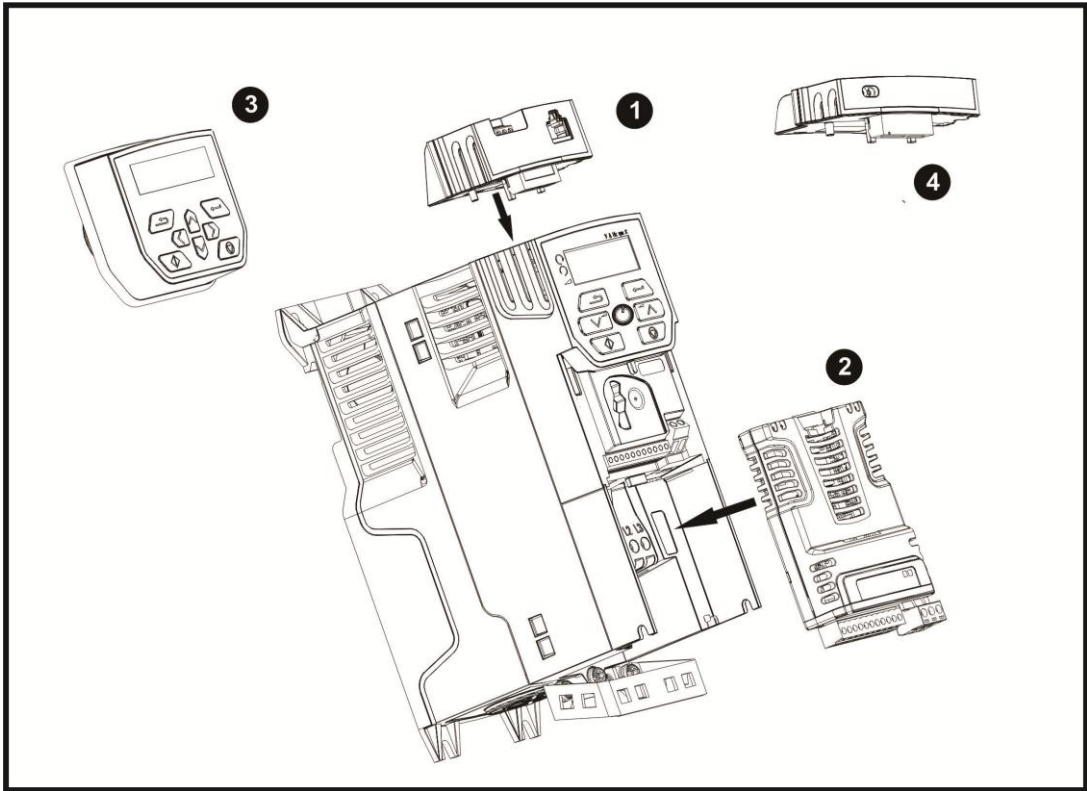
图 2-4 MEV2000 可支持的配件
