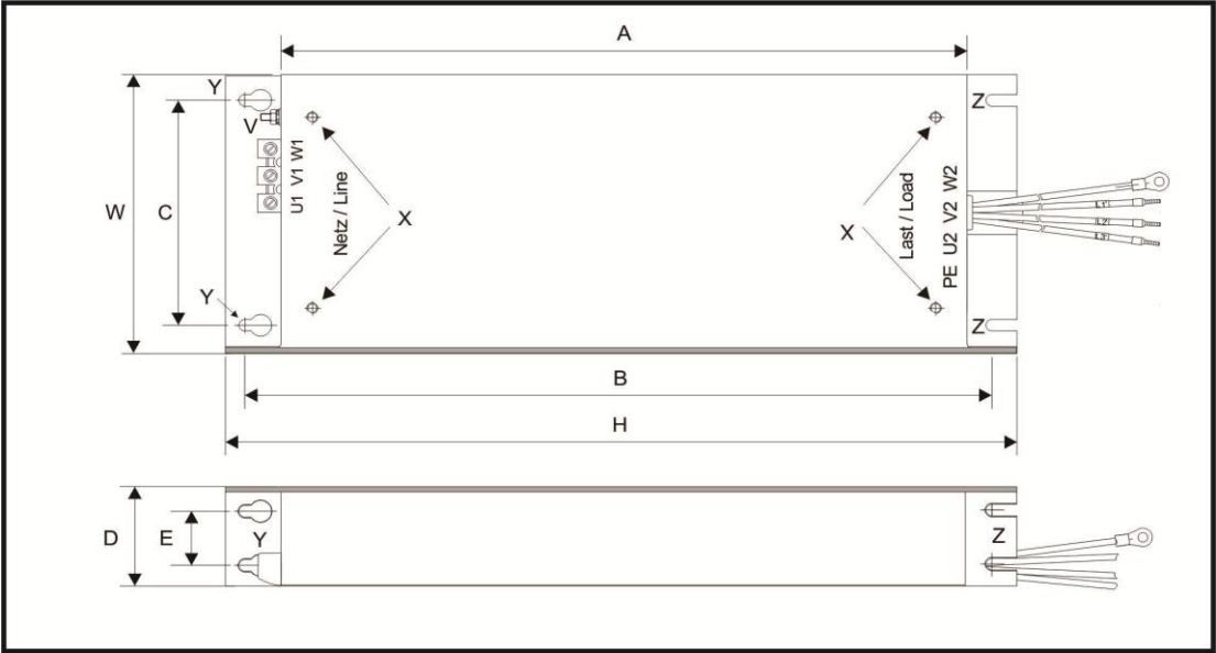
附图 3 EMC 滤波器外形尺寸
