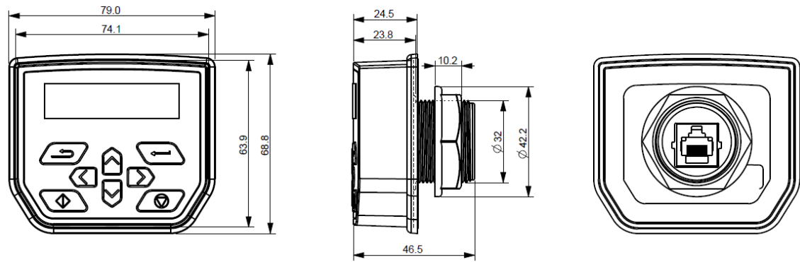
图 2-5 远程键盘尺寸
