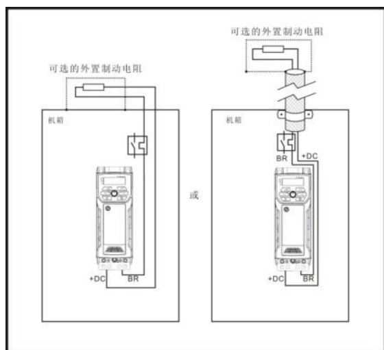
图 3-43 可选外置制动电阻器的屏蔽要求
