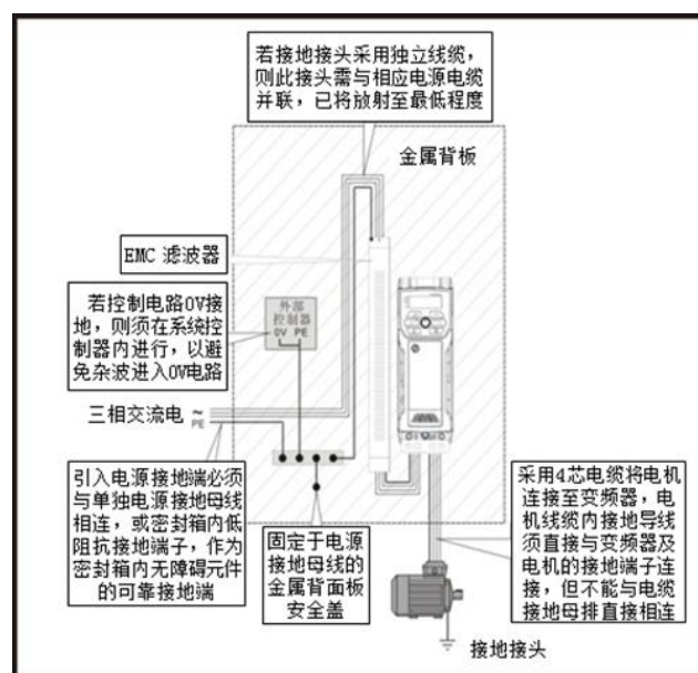
图 3-36 一般 EMC 机壳所示接地连接
