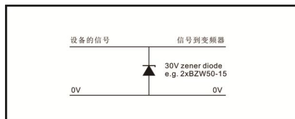
图 3-47 数字及单极输入输出过压抑制
