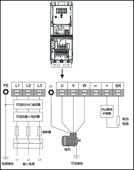
图 3-20 Size2 主回路输入输出连接图
