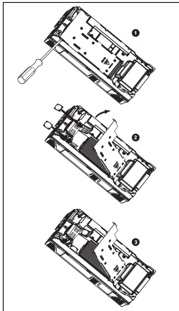
图 3-17 安装 IP 插片
