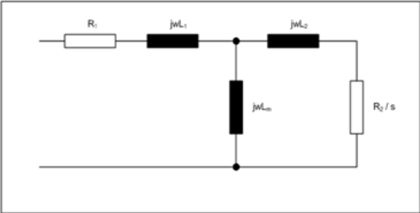
图 5-64 异步电机稳态等效电路图
