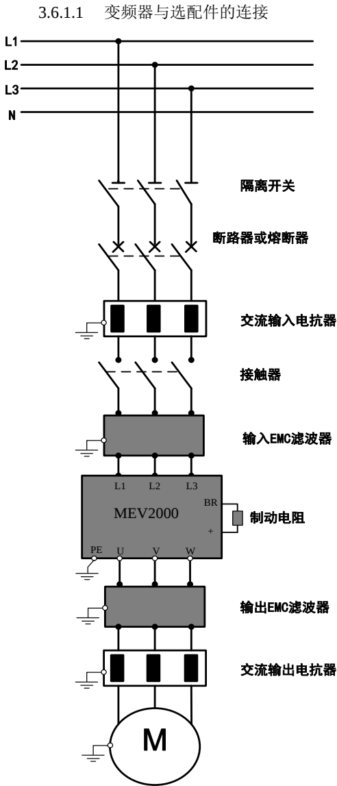
图 3-19 变频器与选配件的连接
