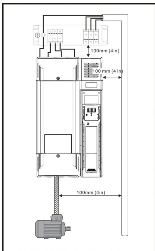
图 3-39 电源及接地线缆间距 (Size7,8)
