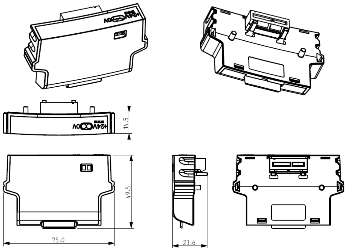
图 2-7 SD 卡适配器尺寸
