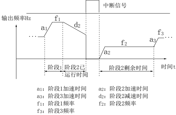
图 5-61 PLC 起动方式 1
