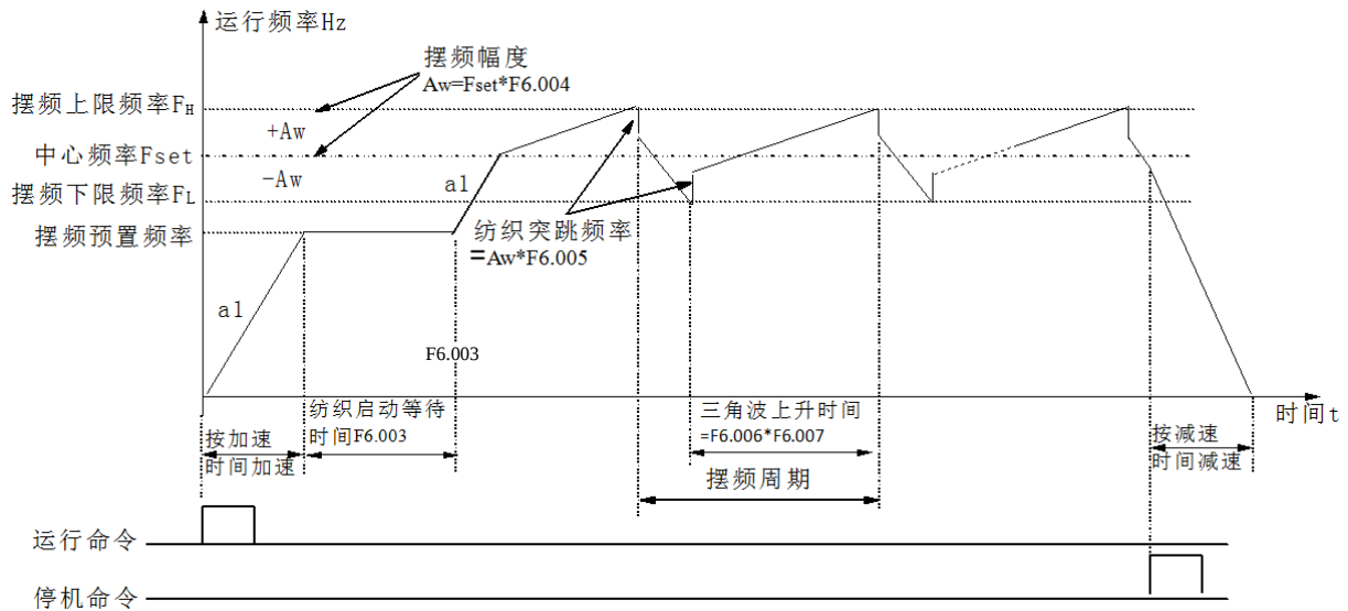
图 5-30 摆频示意图
