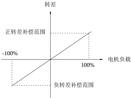
图 5-14 自动转差补偿
