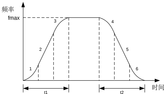
图 5-12 S 曲线加减速
