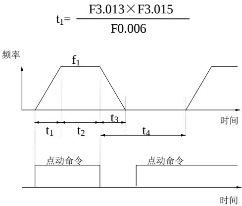
图 5-15 点动运行参数说明
