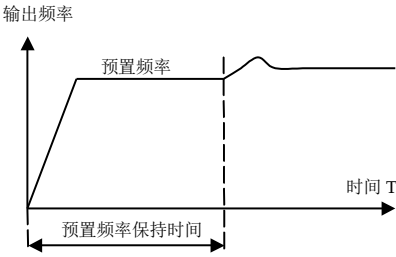
图 5-29 闭环预置频率运行示意图
