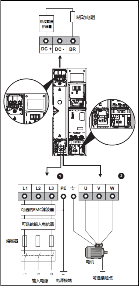
图 3-23 Size5 主回路输入输出连接图
