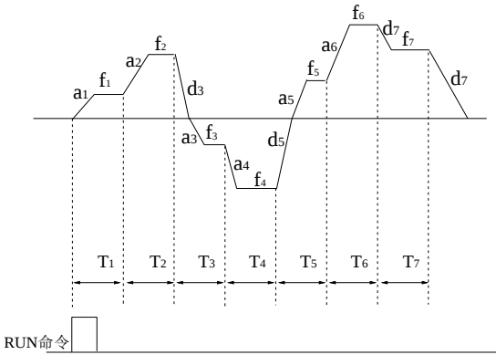
图 5-58 PLC 单循环后停机方式
