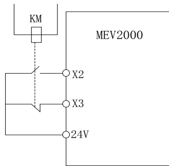
图 5-36 外部设备故障常开/常闭输入示意图
