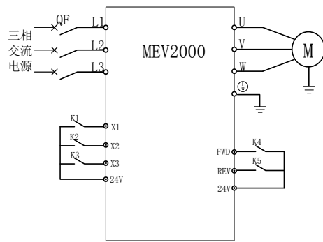
图 5-35 多段速度运行接线图
