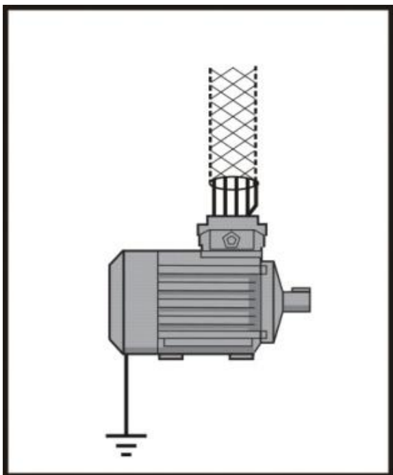
图 3-42 电机电缆屏蔽接地
