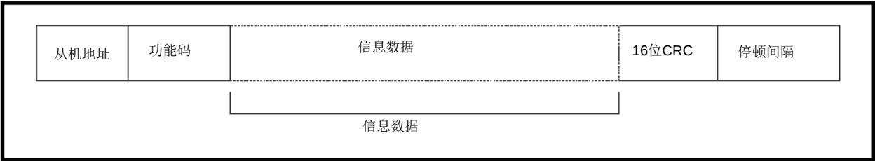
附图 5 帧格式
