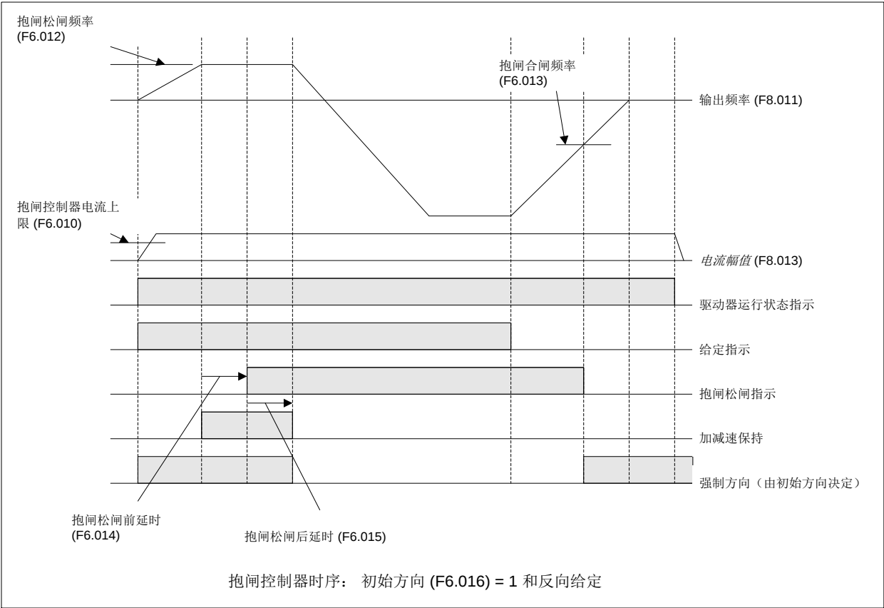
图 5-33 抱闸控制器时序：初始方向 (F6.016) =1 和给定方向
