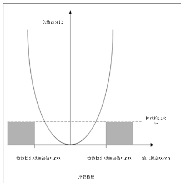
图 5-68 掉载检出示意图
