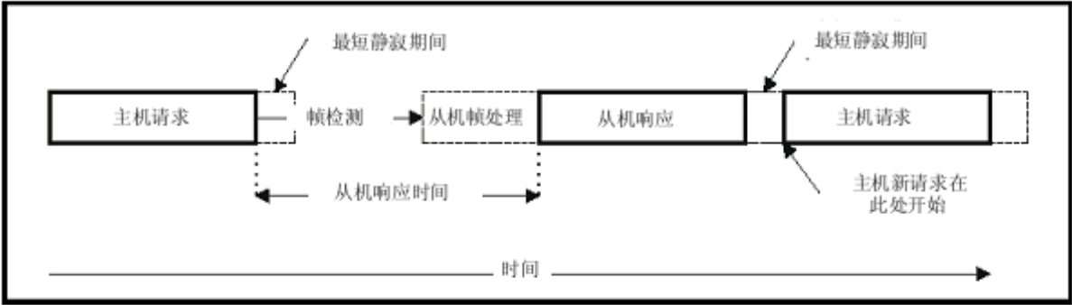
附图 6 主从通讯时间示意图
