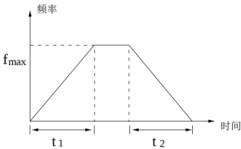
图 5-11 直线加减速
