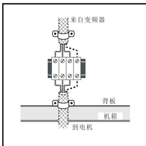
图 3-45 将电机线缆连至柜内接线端子
