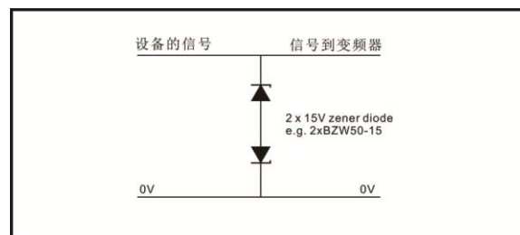
图 3-48 模拟及双极输入输出过压抑制
