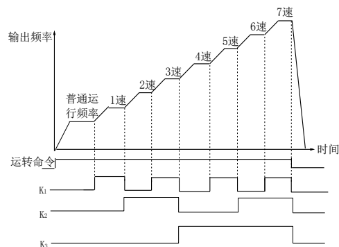
图 5-34 多段速度运行示意图
