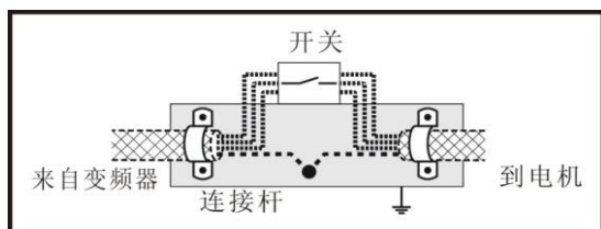
图 3-46 连接电机电缆至隔离开关
