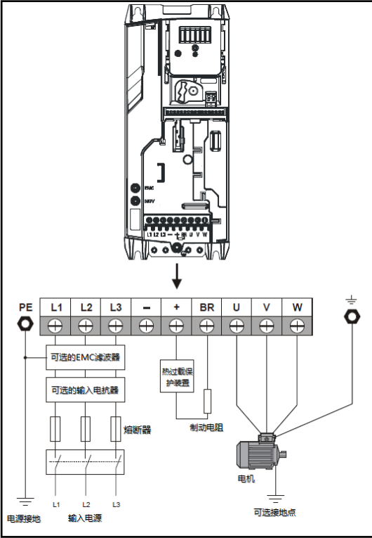
图 3-22 Size4 主回路输入输出连接图
