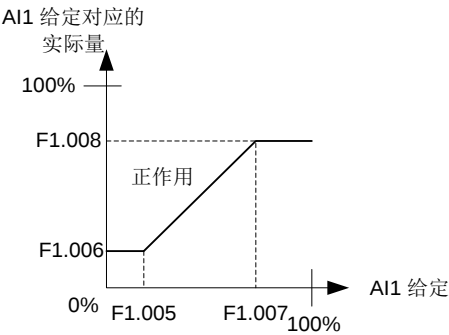
图5-6 模拟输入AI1给定正作用特性
