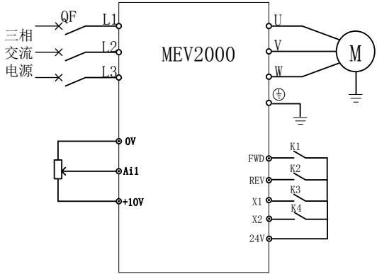
图 5-51 两地控制硬件接线图
