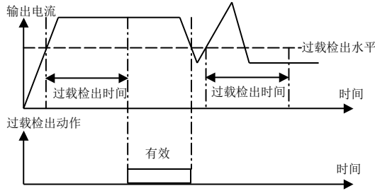
图 5-66 过载预警检出功能示意图
