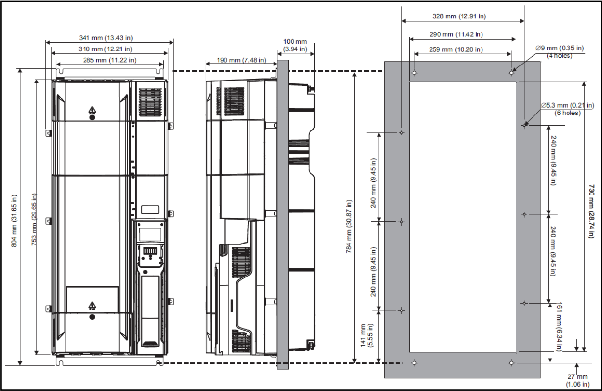
图 3-13 Size8 透壁式安装尺寸图
