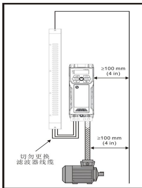
图 3-38 电源及接地线缆间距（Size2-6）
