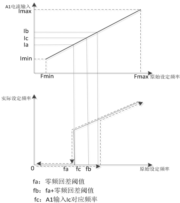
图 5-54 零频回差运行
