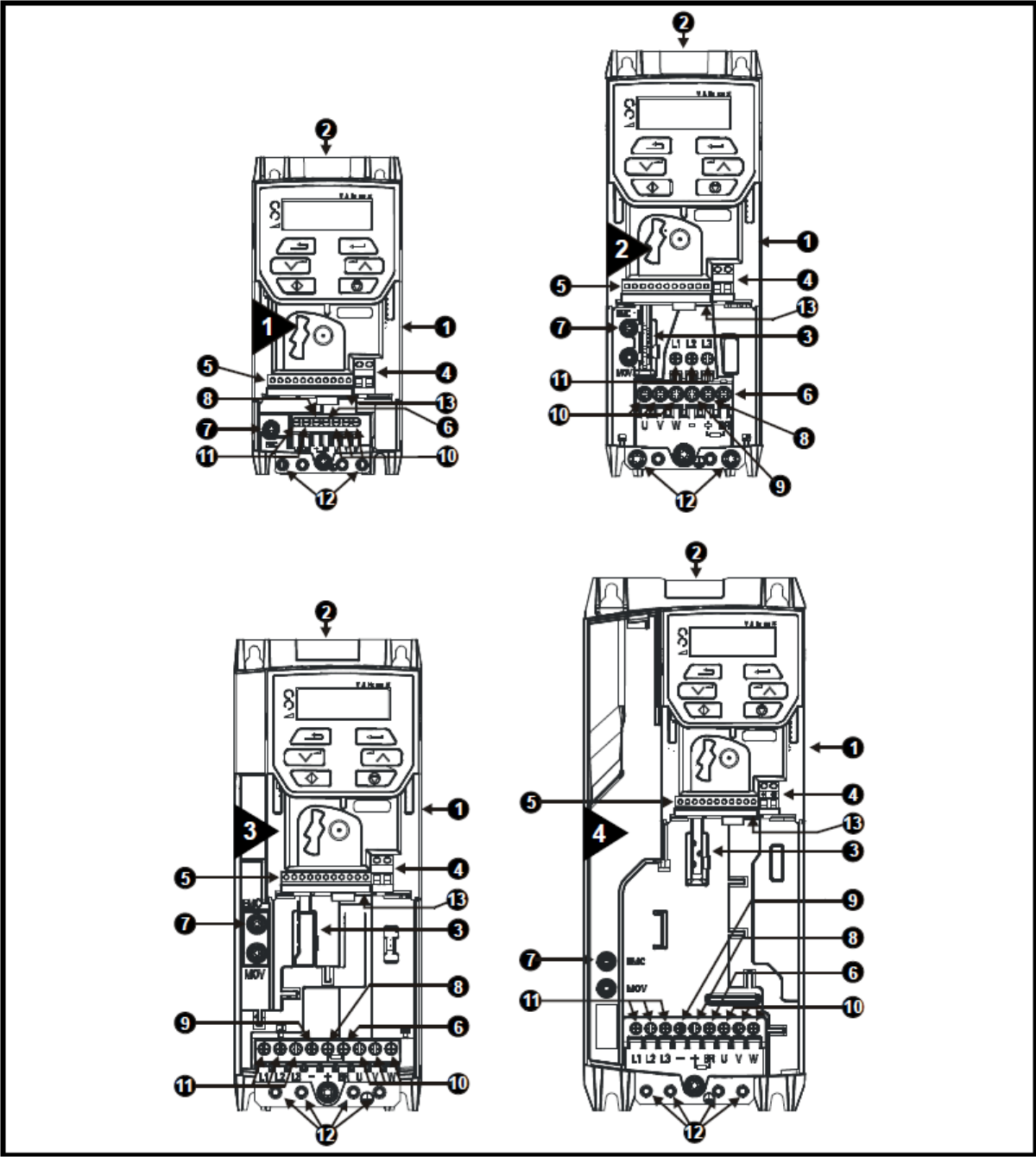
图 2-1 Size 2~4 变频器各部位名称示意图
