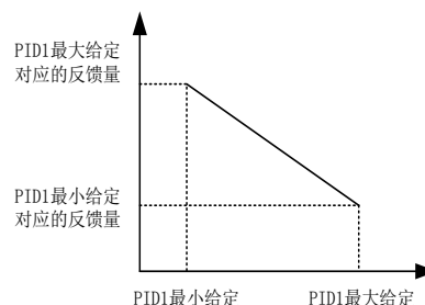
图 5-27 给定、反馈曲线示意图
