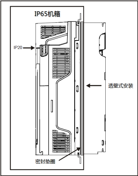
图 3-14 IP65 等级的柜内安装图
