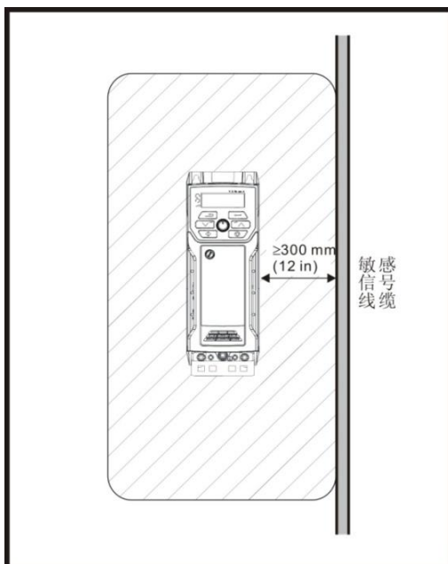
图 3-40 敏感信号电路间距
