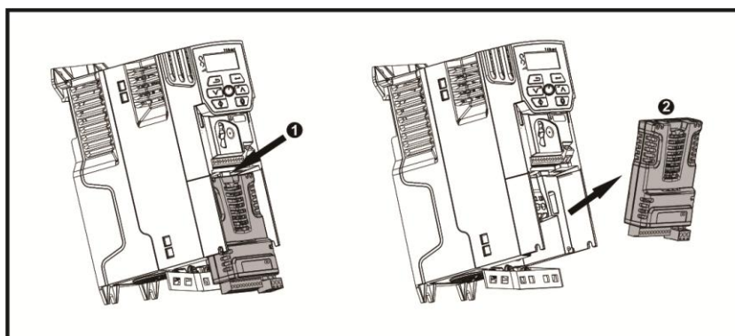
图 3-6 选件卡拆卸示意图
