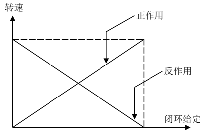
图 5-26 闭环调节特性示意图
