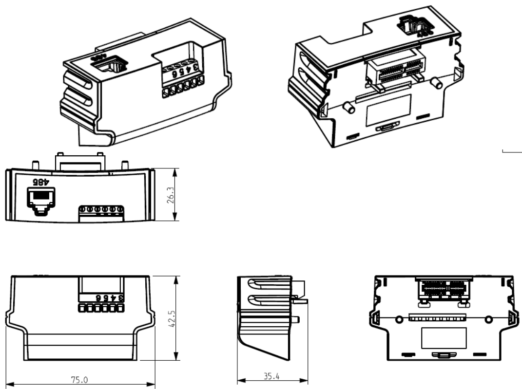
图 2-6 外置 RS485 适配器尺寸
