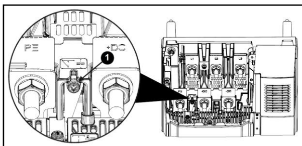
图 3-35 Size7-8 内置 EMC 滤波器移除示意图
