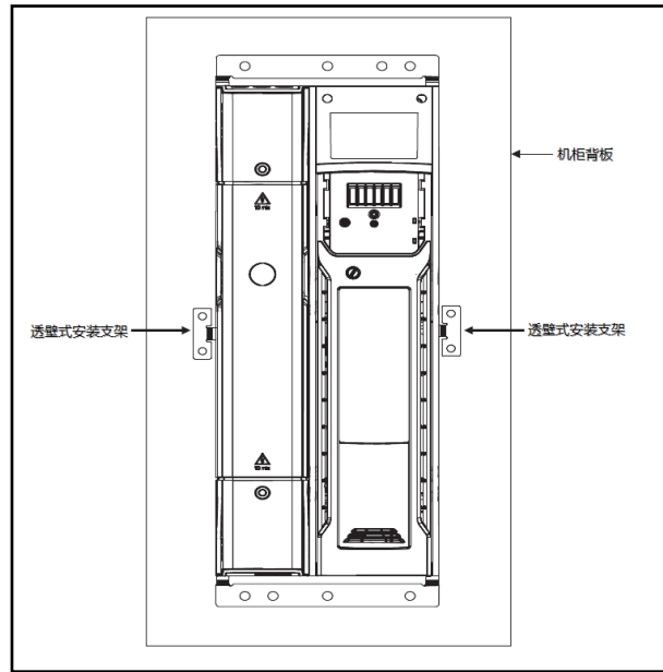
图 3-16 透壁式安装示意图
