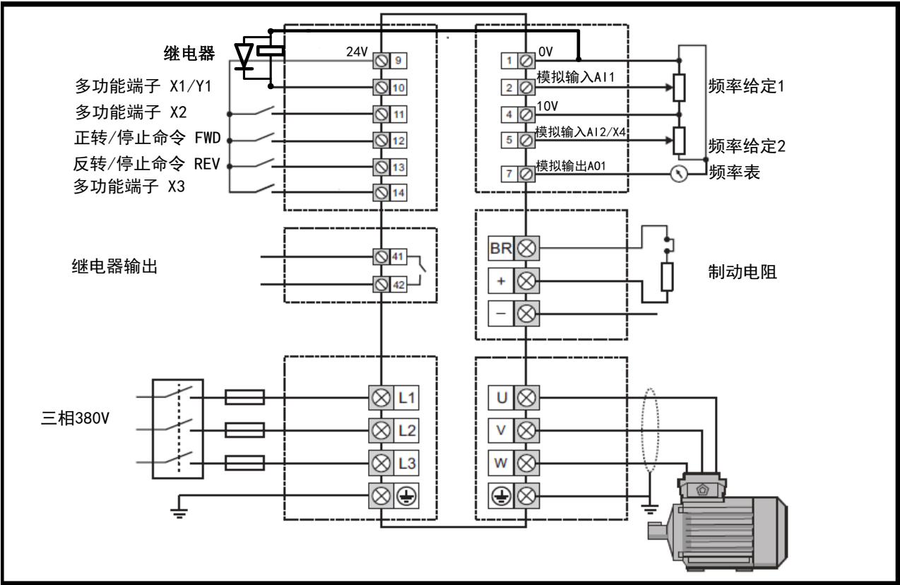
图 3-26 端子连接图
