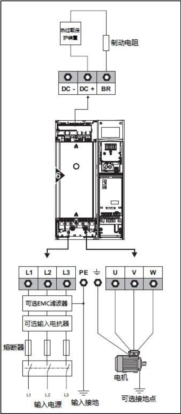
图 3-24 Size6 主回路输入输出连接图
