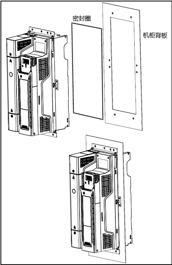
图 3-15 安装密封圈
