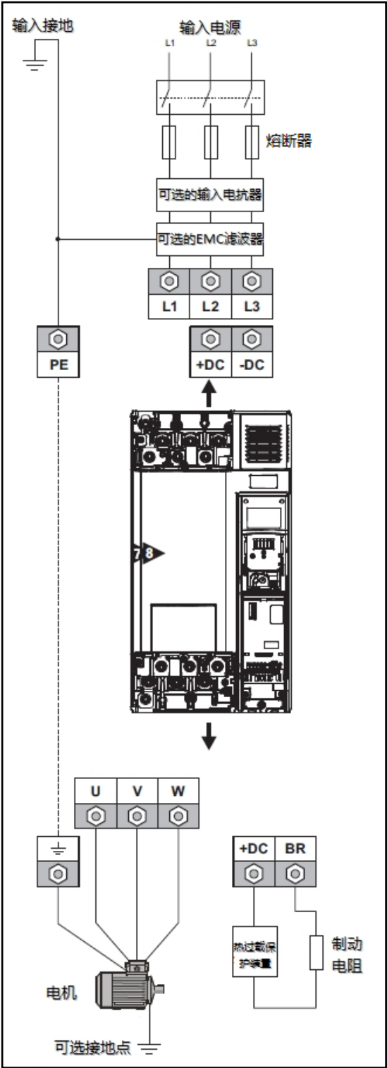
图 3-25 Size7-8 主回路输入输出连接图
