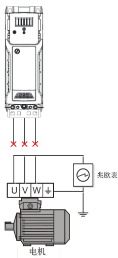
图 1-1 电机绝缘检查示意图
