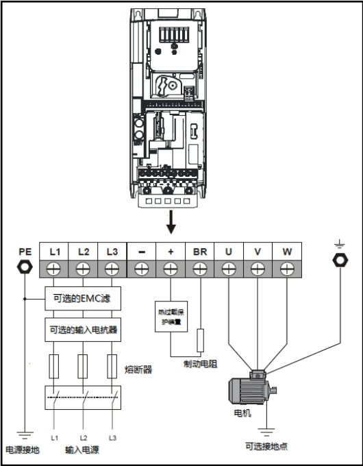
图 3-21 Size3 主回路输入输出连接图
