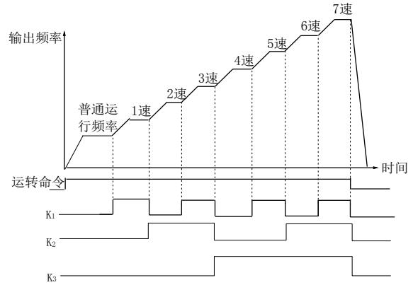
图 5-29 多段速度运行示意图
