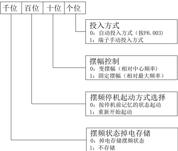
图 5-26 摆频运行方式参数含义
