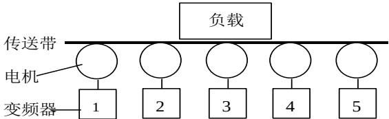
图 5-47 下垂控制示意图
