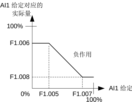
图 5-7 模拟输入 AI1 给定反作用特性
