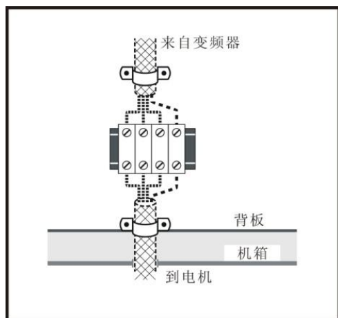
图 3-338 将电机线缆连至柜内接线端子
