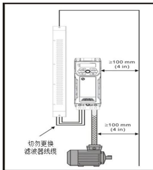
图 3-272 电源及接地线缆间距（Size1-6）
