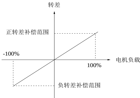
图 5-14 自动转差补偿
