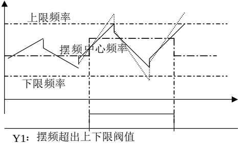
图 5-32 摆频幅度限制
