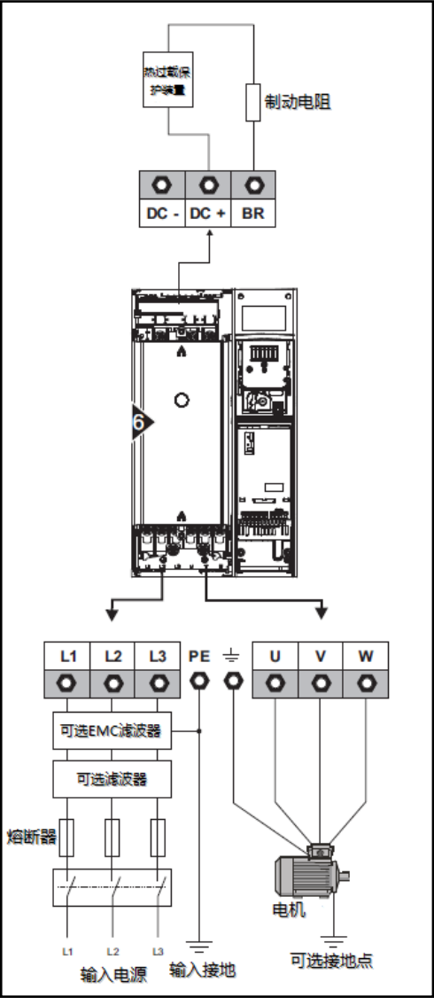
图3-20 Size6主回路输入输出连接图
