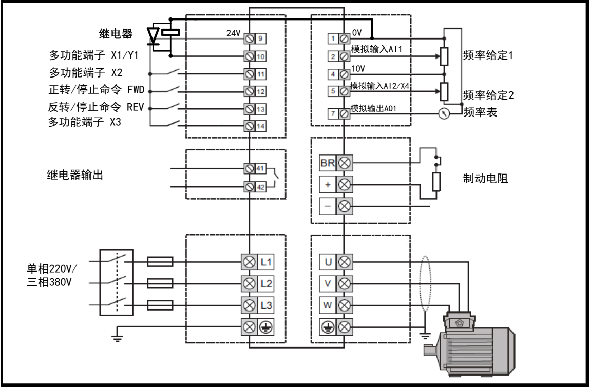
图 3-182 端子连接图
