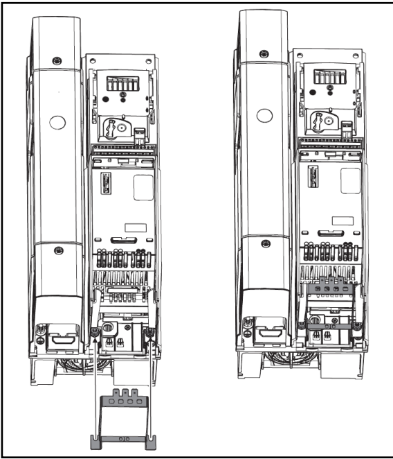
图 3-204 Size5-7 接地支架安装示意图（size5 为例）
