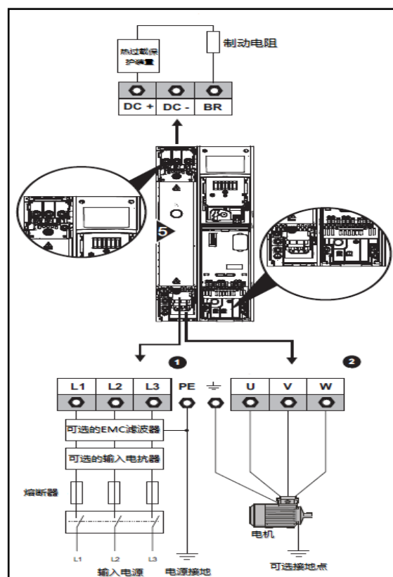
图 3-169 Size5 主回路输入输出连接图
