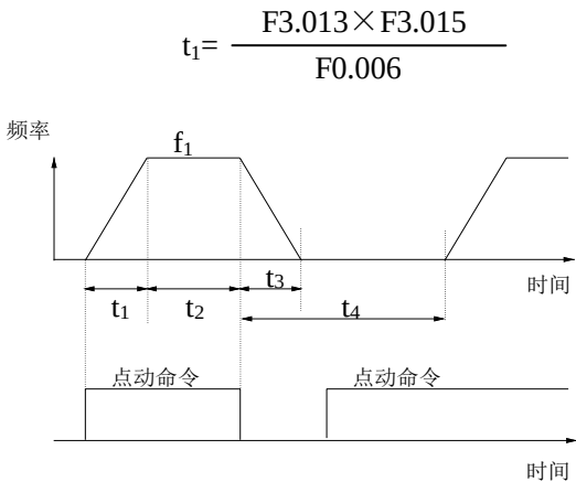
图 5-15 点动运行参数说明
