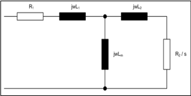
图 5-59 异步电机稳态等效电路图 稳态参数被转化为等效的瞬态模型参数。
