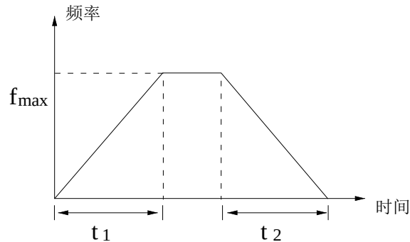
图 5-11 直线加减速
