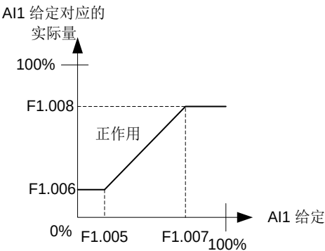
图 5-6 模拟输入 AI1 给定正作用特性
