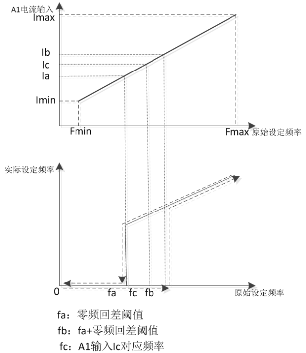
图 5-49 零频回差运行
