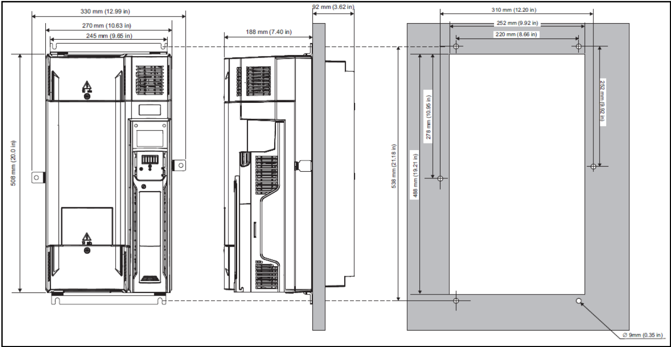
图3-8 Size7透壁式安装尺寸图
