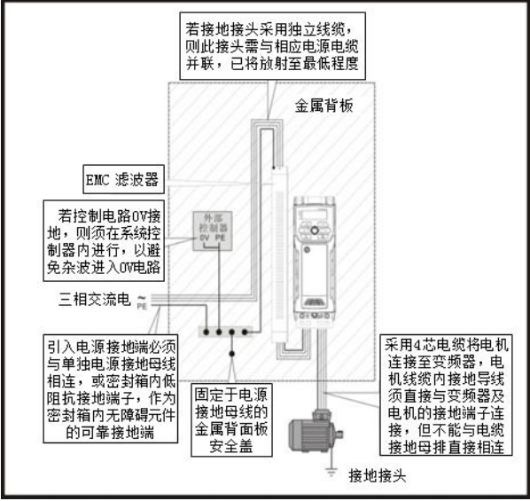
图 3-30 一般 EMC 机壳所示接地连接
