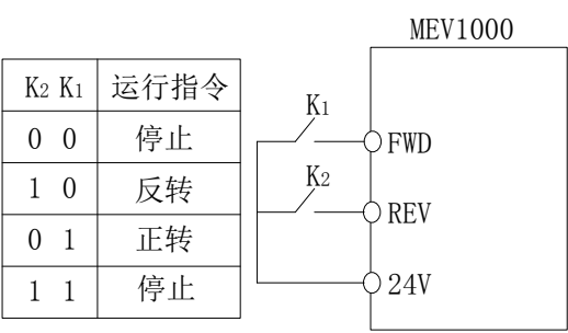
图 5-33 两线式运转模式 1
