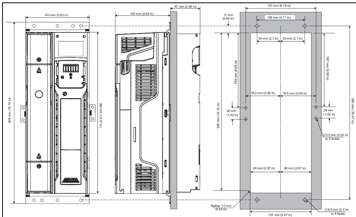
图 3-6 Size5 透壁式安装尺寸图
