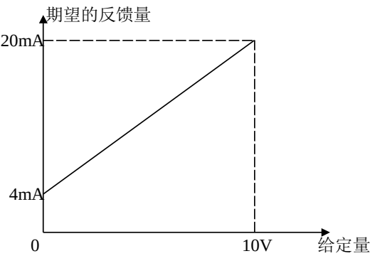
图5-20 给定量和期望反馈量
