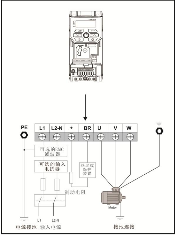
图 3-125 Size1 主回路输入输出连接图
