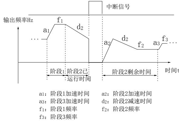
图 5-57 PLC 起动方式 2
