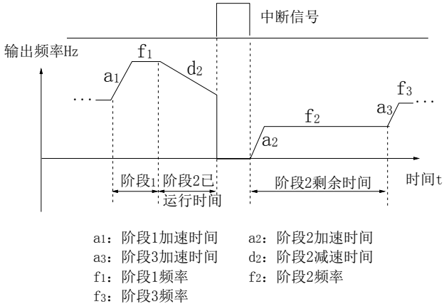
图 5-56 PLC 起动方式 1
