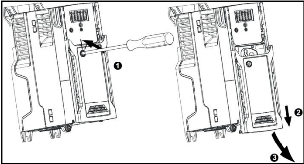
图 3-2 size1～ 4 盖板拆卸示意图
