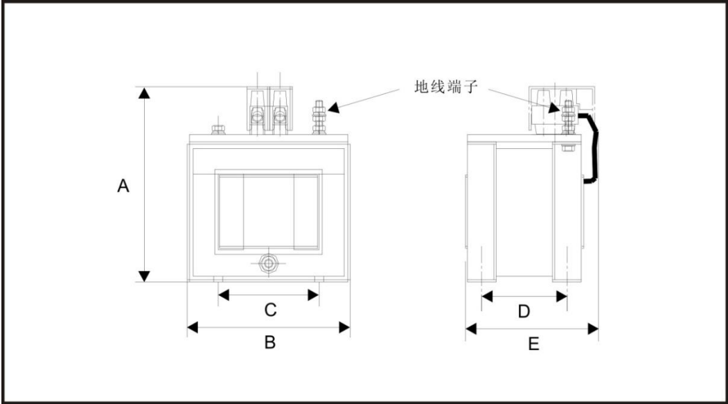
附图 1 交流输入电抗器外形图
