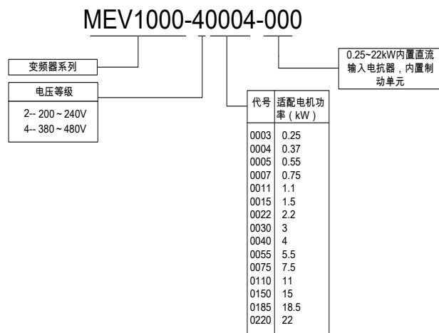
图 A-1 变频器型号说明
