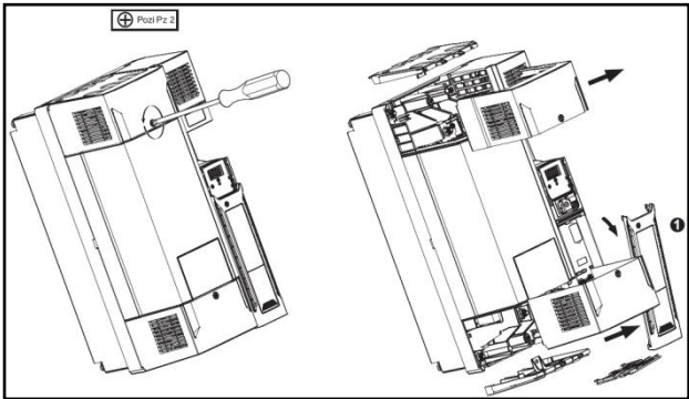
图 3-3 size5～7 盖板拆卸示意图
