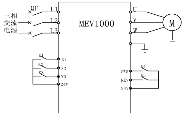
图 5-30 多段速度运行接线图
