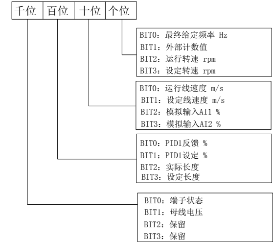
图 5-43 LED 停机显示参数选择设定
