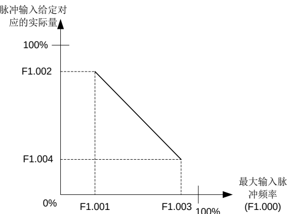
图5-4 端子脉冲给定正作用特性
