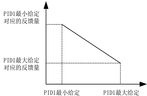
图 5-22 给定、反馈曲线示意图
