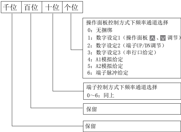
图 5-44 运行命令通道捆绑频率给定通道
