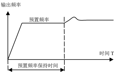
图 5-24 闭环预置频率运行示意图
