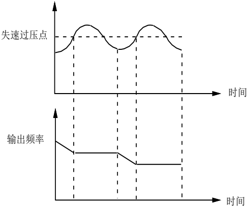
图 5-60 过压失速功能
