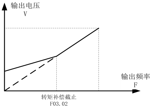
图 6-4 转矩补偿图
