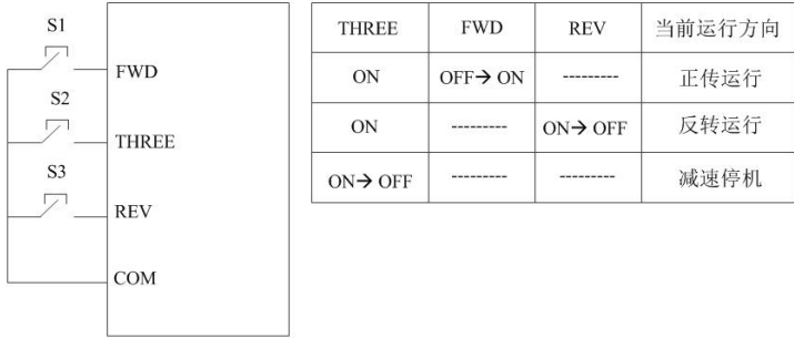
图 6-10 三线式控制 2
