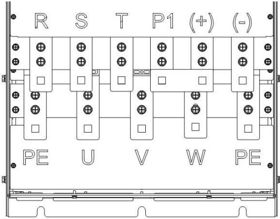
图 3-6 KV300-T6-160KW~KV300-T6-220KW 主回路接线端子图
