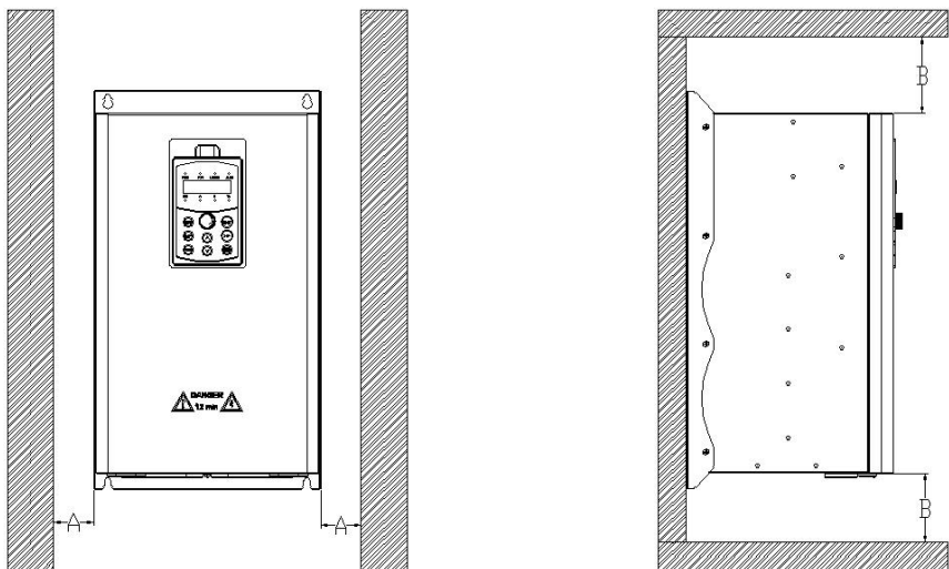
图 3-1 KV300-T6-22KW 及以上功率等级的安装方向和距离要求
