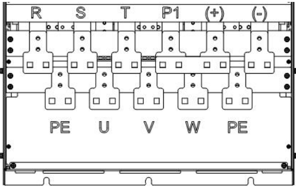
图 3-7 KV300-T6-250KW~KV300-T6-630KW 主回路接线端子图
