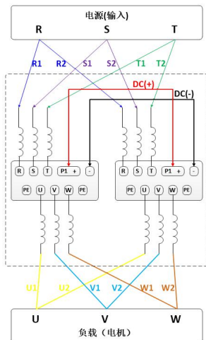
图 3-15 630KW（并机）变频器主回路连接说明
