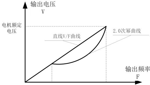
图 6-3 V/F 曲线图
