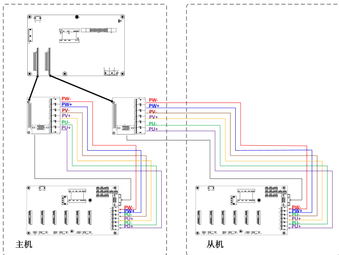
图 3-14 630KW~1MW（并机）变频器弱电部分连接说明
