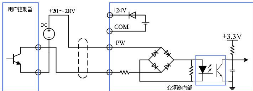
图 3-22 NPN 型灌电流接线方式
