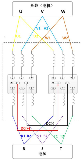
图 3-16 700KW~1MW (并机) 变频器主回路连接说明
