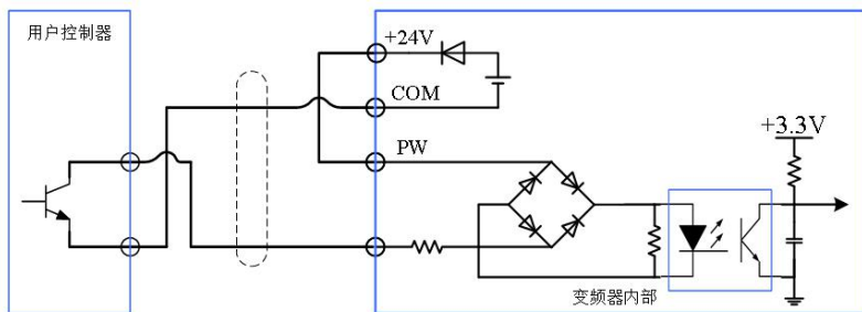
图 3-20 NPN 型灌电流接线方式
