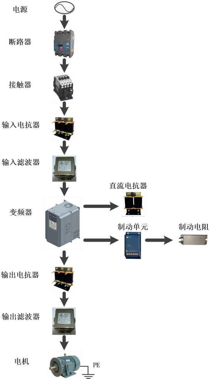
图 3-3 产品外围元器件的标准配置图
