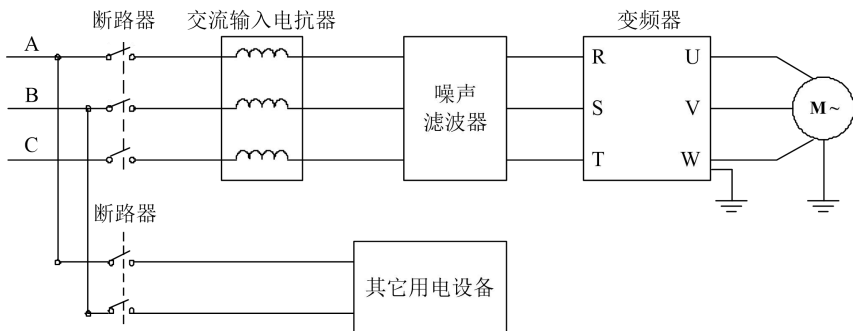
图 3-10 主回路电源侧连接图
