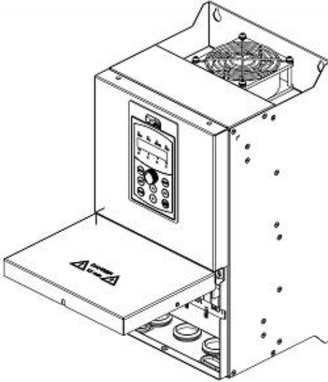
图 3-2 KV300-T6-22KW~ KV300-T6-355KW 盖板安装与拆卸图
