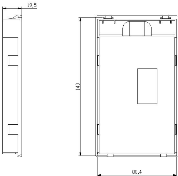
图 2-5 外引键盘支架外形尺寸图(单位 mm)
