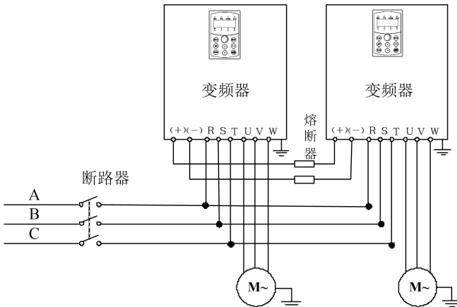
图 3-13 共直流母线的连接
