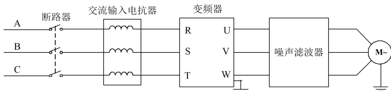
图 3-11 主回路电机侧连接图
