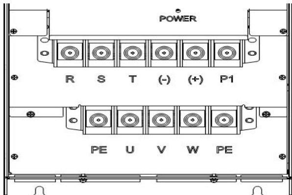
图 3-5 KV300-T6-55KW~KV300-T6-132KW 主回路接线端子图
