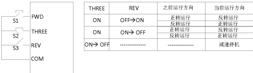
图 6-9 三线式控制 1
