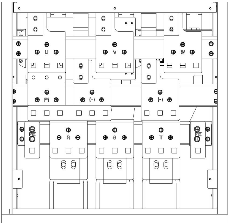
图 3-8 KV300-T6-400KW~KV300-T6-630KW 主回路接线端子图
