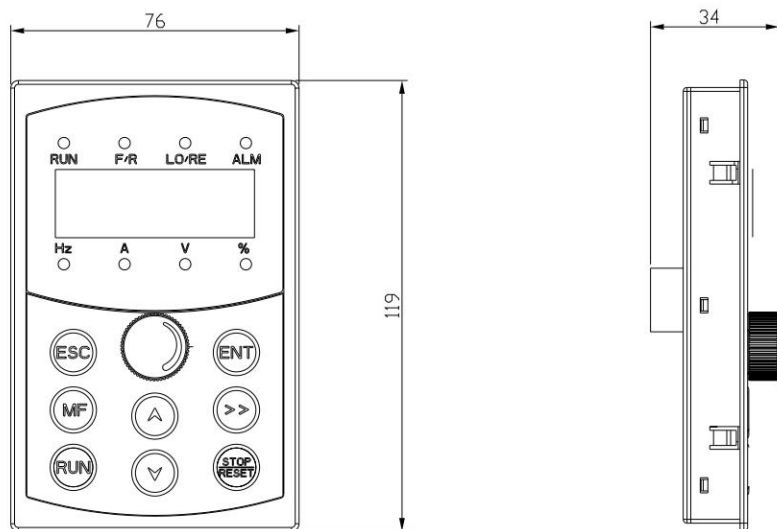
图 2-4 面板外形及尺寸图(单位: mm)
