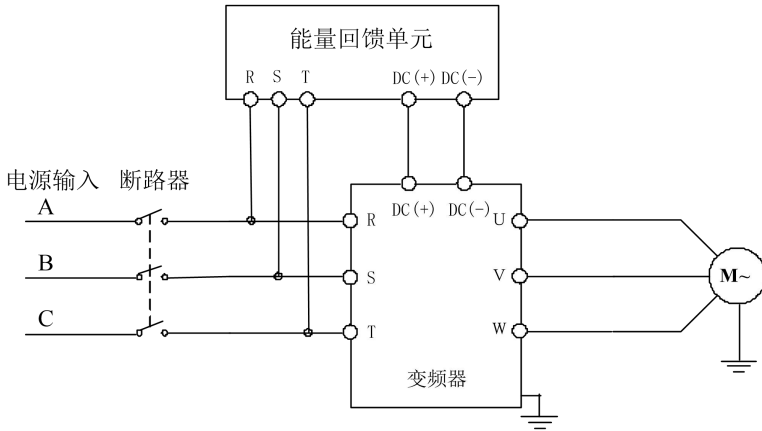
图 3-12 能量回馈单元连接图
