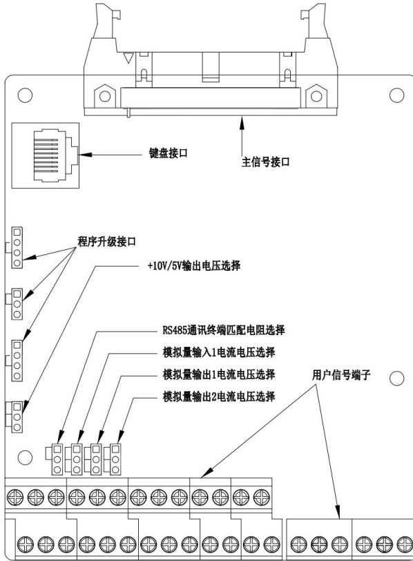
图 3-17 控制板示意图
