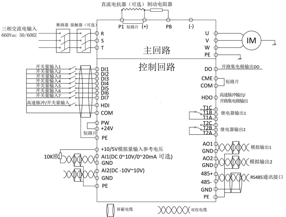
图 3-9 标准接线图
