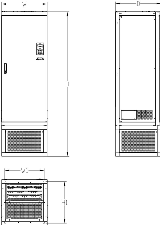
d) 适用于, KV300-T6-400KW ~ KV300-T6-630KW
