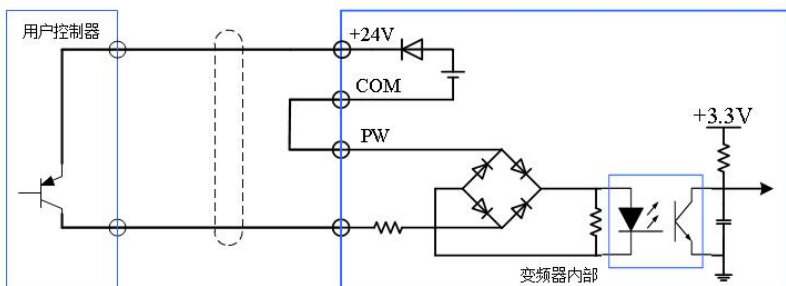
图 3-21 PNP 型拉电流接线方式
