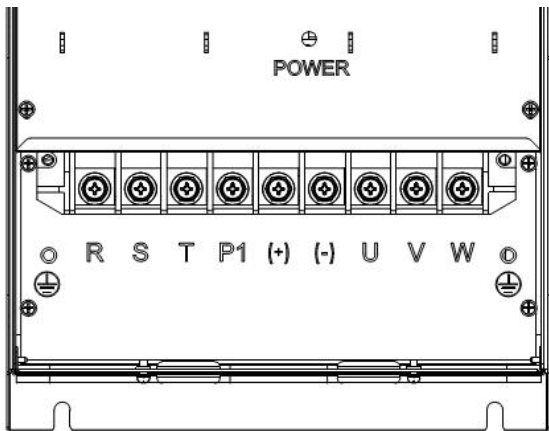
图 3-4 KV300-T6-22KW~KV300-T6-45KW 主回路接线端子图
