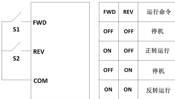
图 6-8 两线式控制 2
