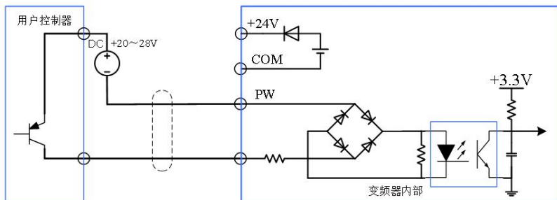
图 3-23 PNP 型拉电流接线方式
