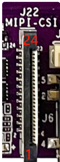
J22 24Pin FPC座 0.5mm 垂直抽拉式 单面触点 引脚定义说明
