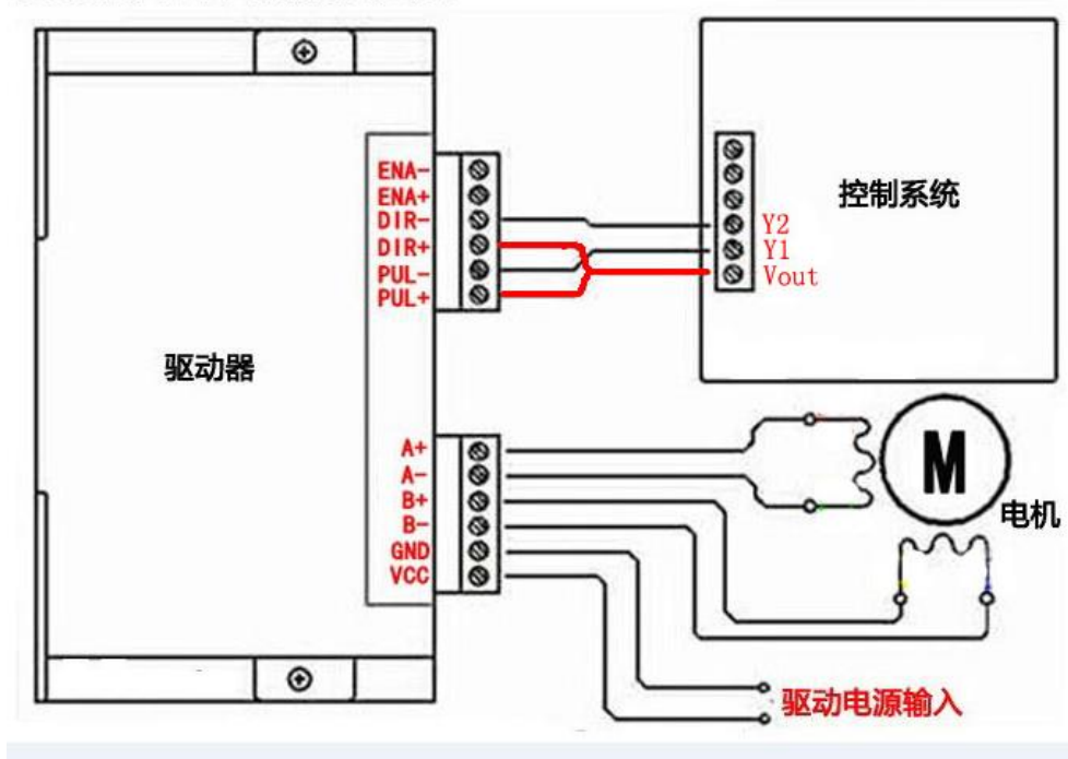
系统接线图（以共阳极接法为例）
