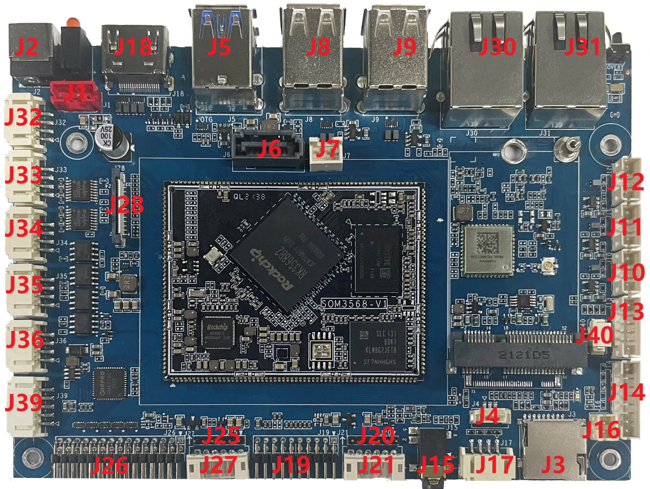
图4. IDO-EVB3568-V1正面接口位号图
