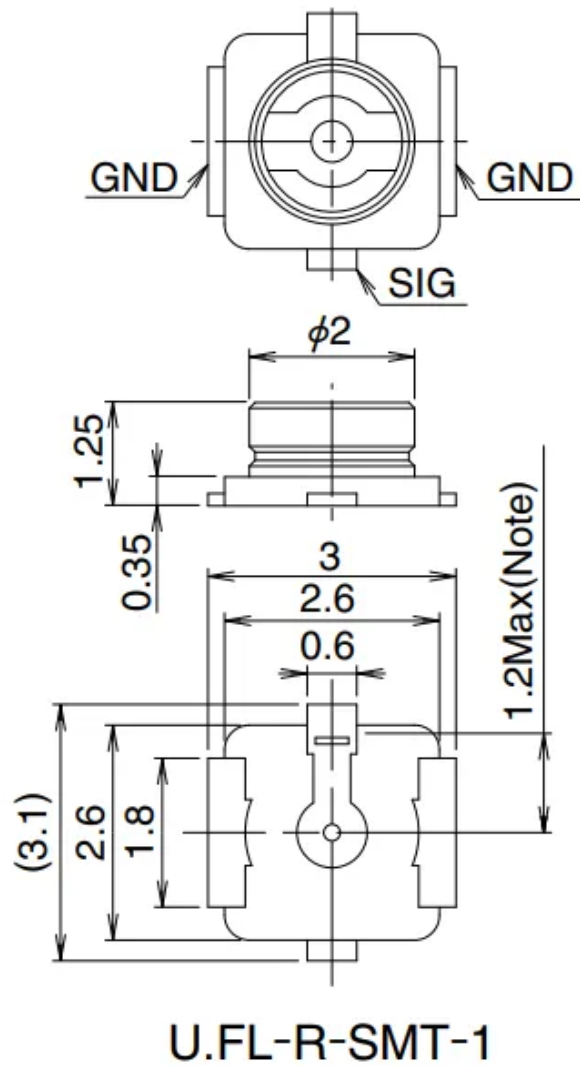
图15. IDO-EVB3568-V1 IPEX天线座示意图
