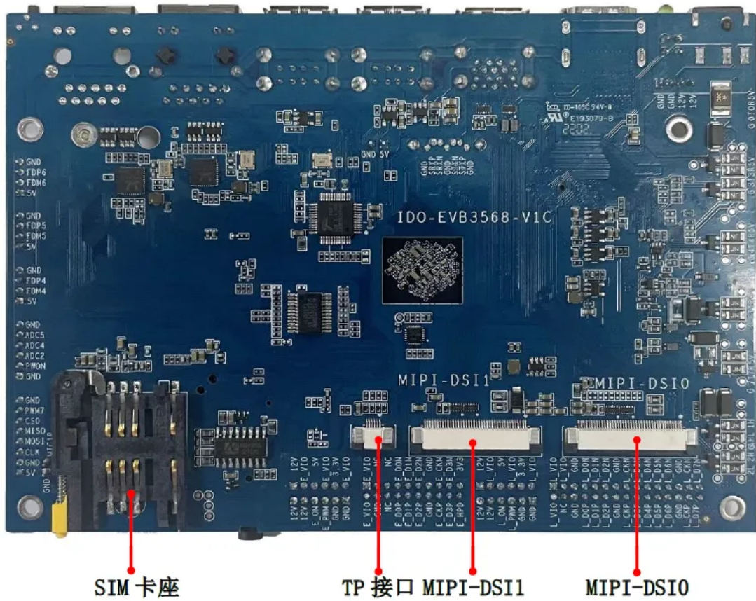
图2. IDO-EVB3568-V1反面接口图
