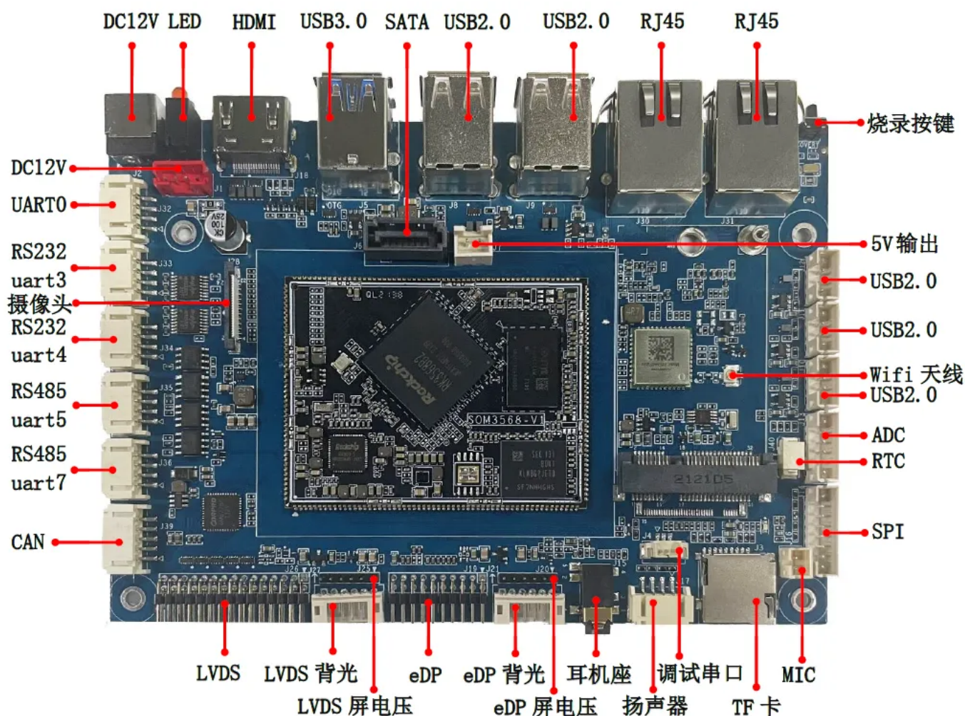
图1. IDO-EVB3568-V1正面接口图
