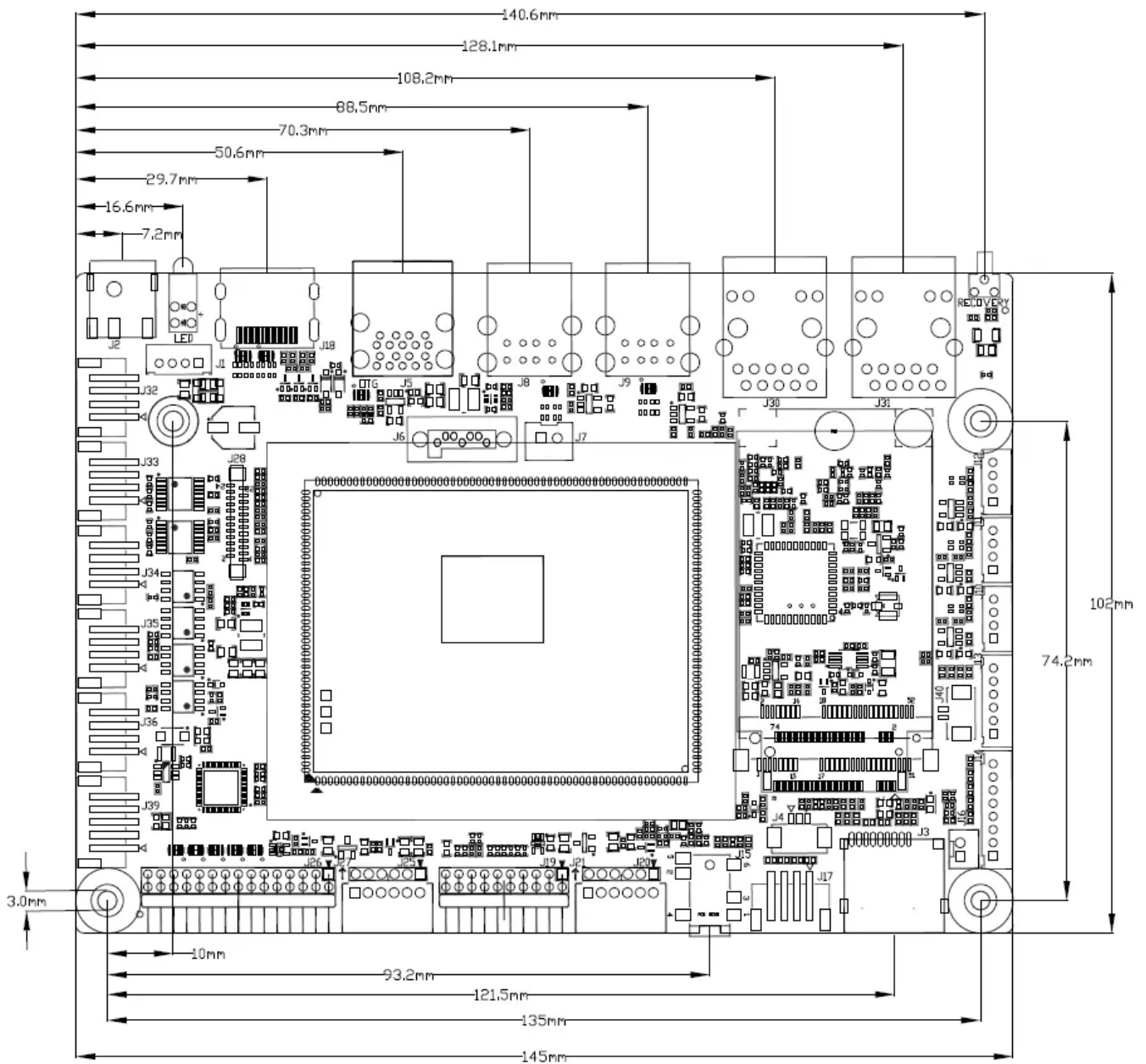
图3. IDO-EVB3568-V1尺寸图
