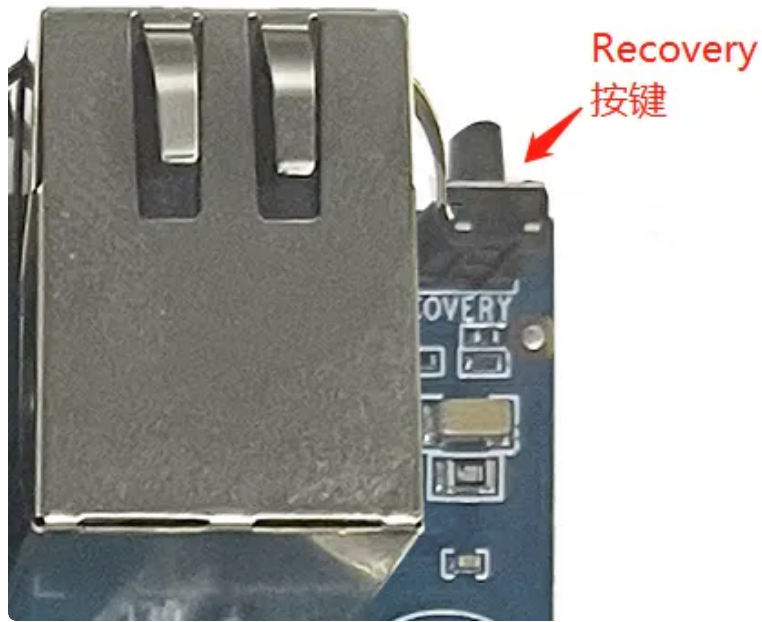
图12. IDO-EVB3568-V1 烧录按键
