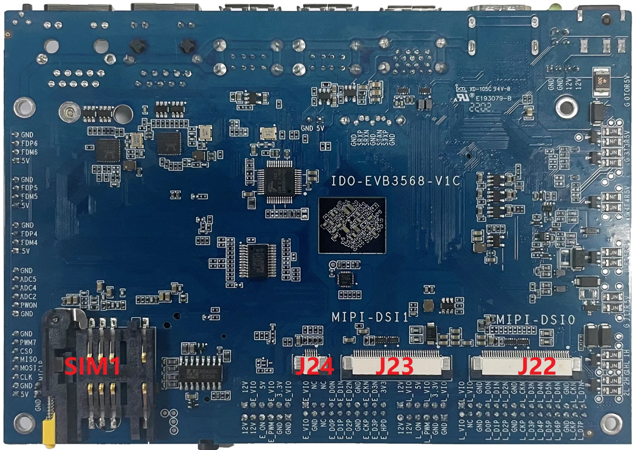
图5. IDO-EVB3568-V1反面接口位号图
