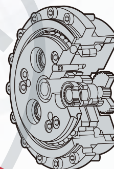
精密减速机
